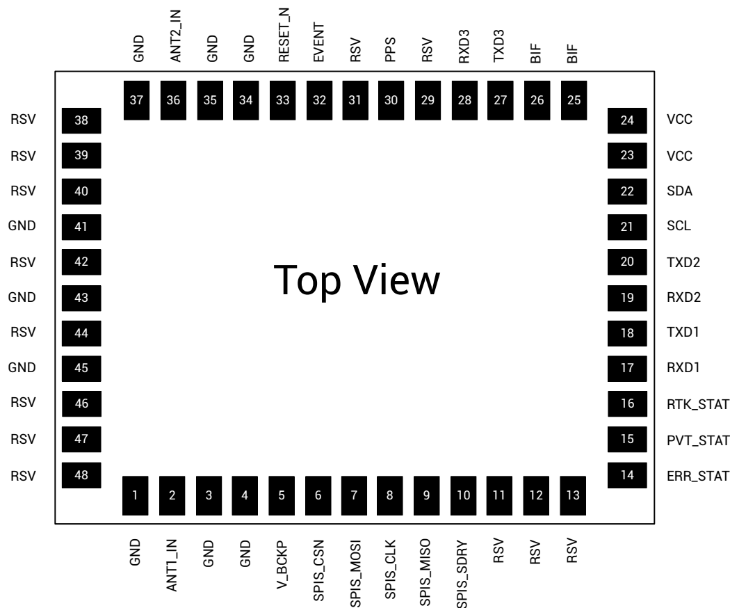
图 2-1 引脚图
