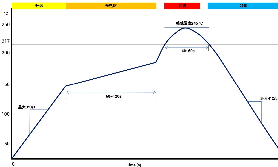
图 4-1 焊接温度曲线图（无铅）
