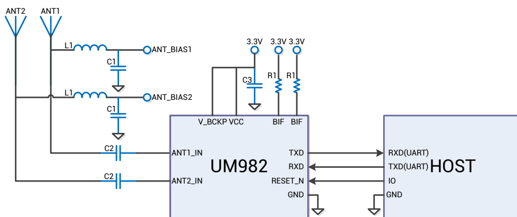
图 3-1 最小系统推荐设计
