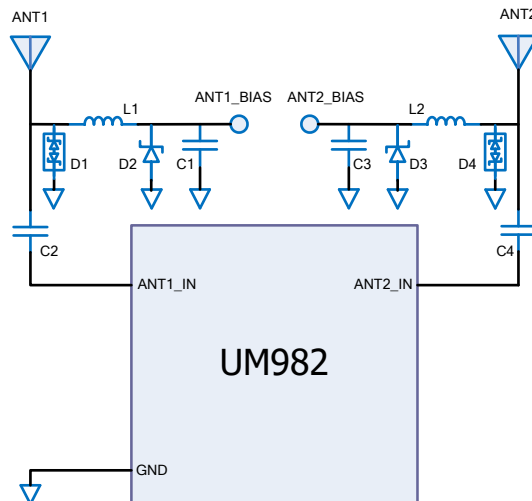
图 3-2 外部天线馈电参考电路图
