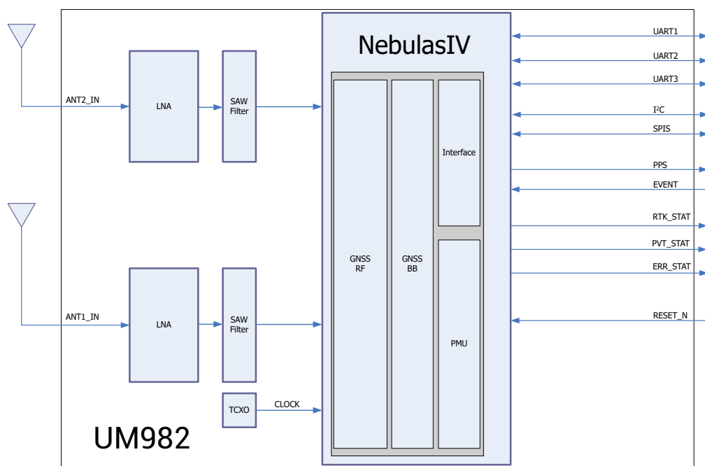
图 1-2 功能框图
