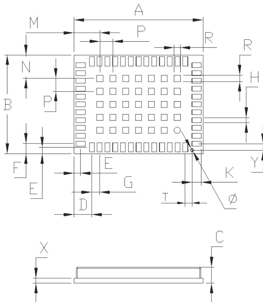
图 2-2 机械尺寸
