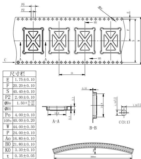
图 5-3 卷装示意图
