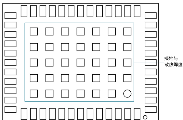
图 3-3 接地与散热焊盘（底视图）
