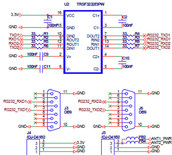
图 3-2 UM4B0 参考设计
