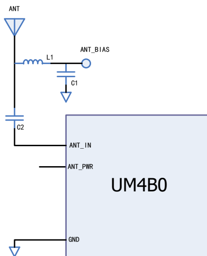
图 3-6 UM4B0 外部天线馈电参考电路
