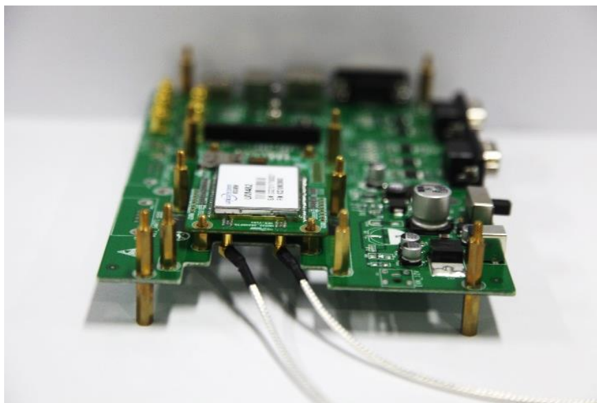
图 4-3 连接天线
