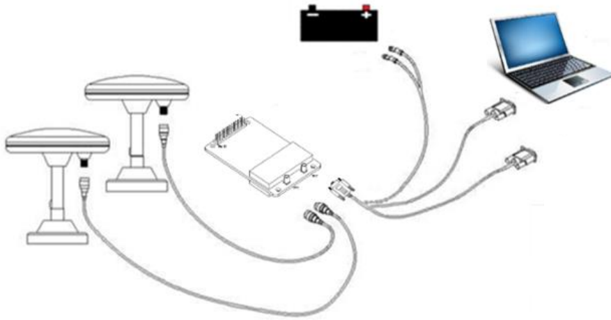
图 4-1 连接示意图
