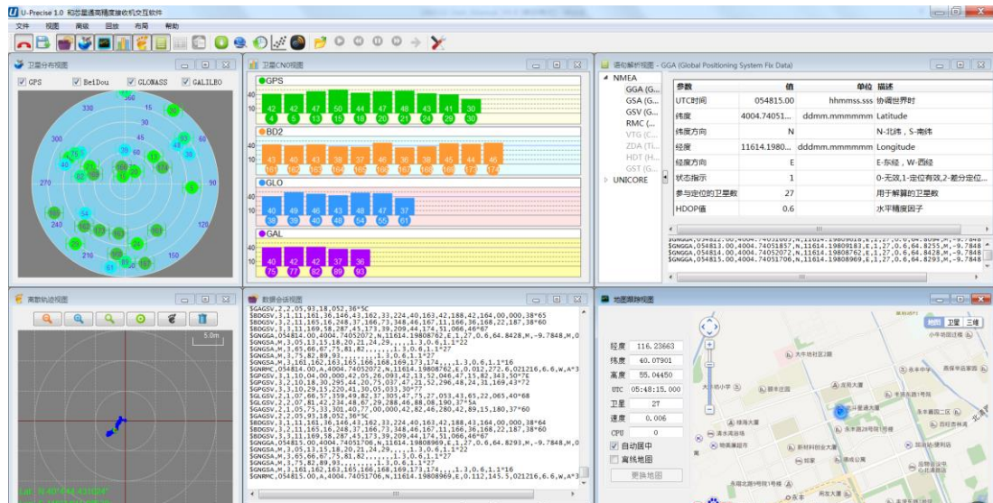
图 4-5 Uprecise 界面
