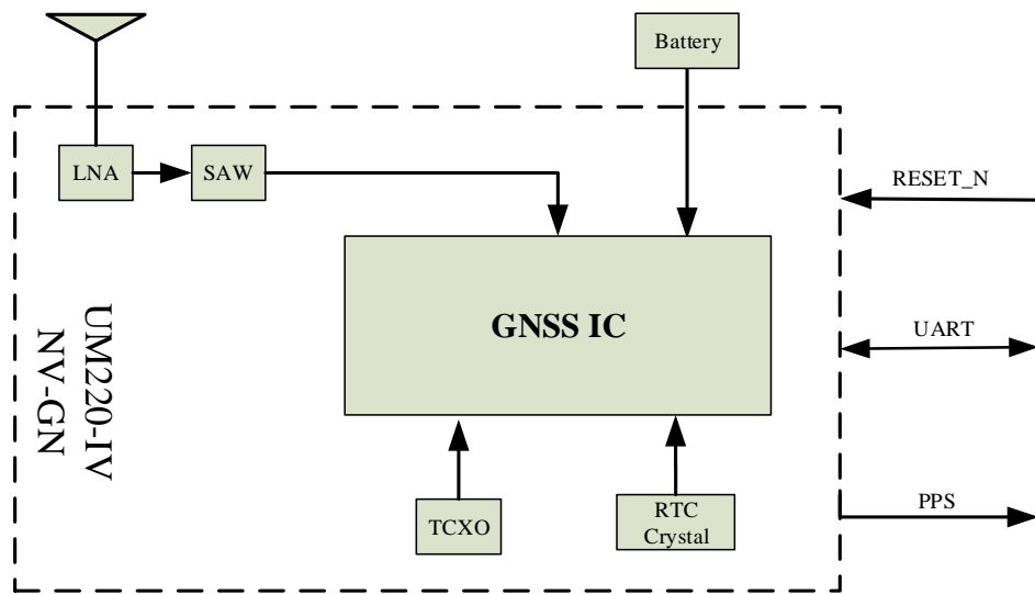
图 1-2 结构框图
