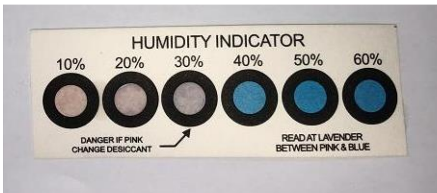
图 6-3 湿度卡的 30%标识圈显示为粉红色
