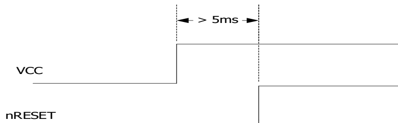
图 4-1 UM220-IV NV-GN 模块复位信号
