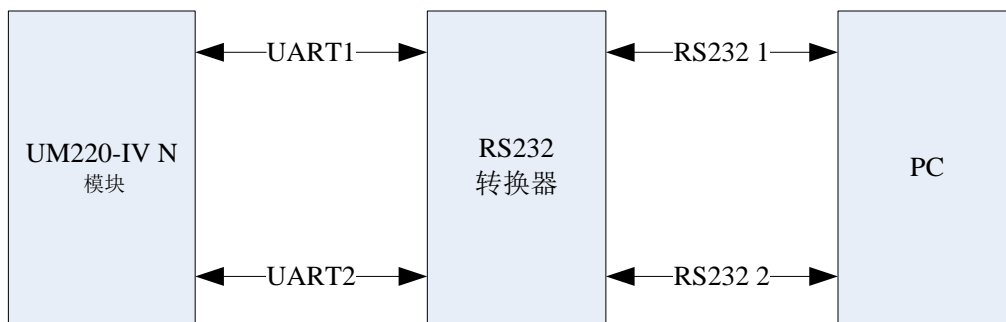
图 4-4 串口连接到 PC
