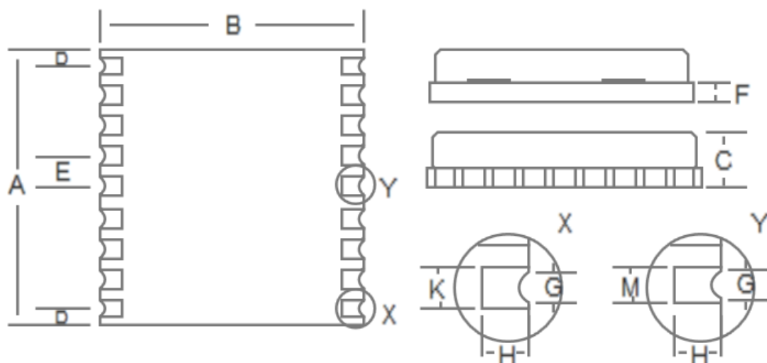
图 3-1 机械图
