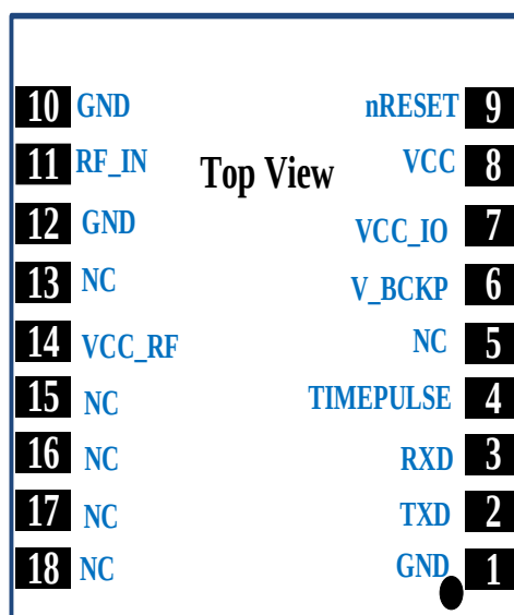
图 3-2 UM220-IV M0 管脚图
