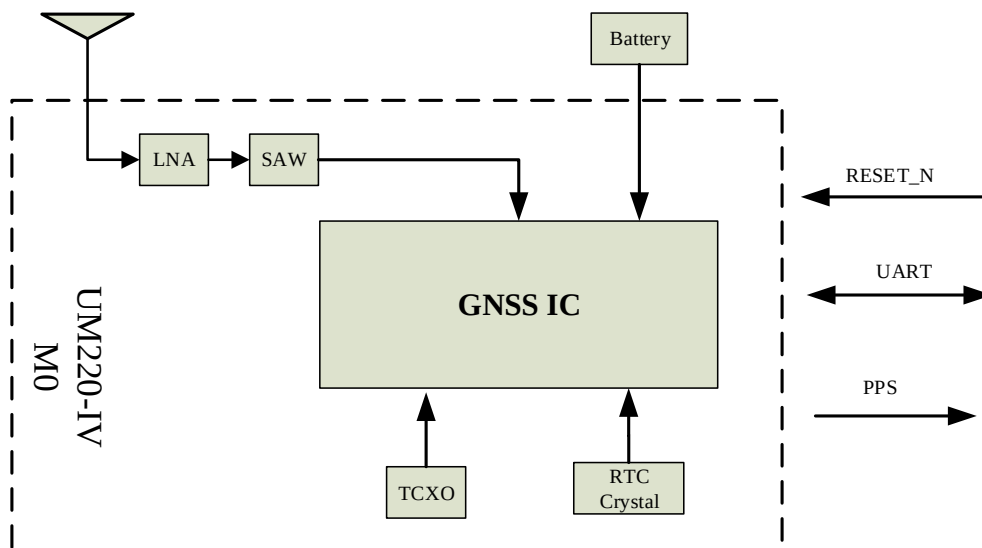
图 1-2 结构框图
