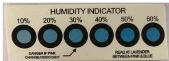
图 6-2 湿度卡的 30%标识圈显示为蓝色
