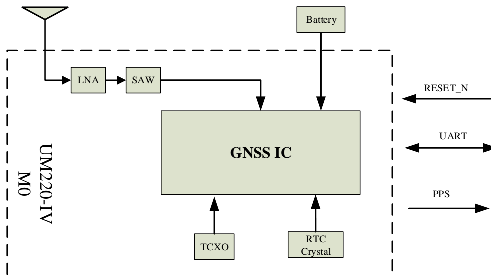
图 1-2 结构框图
