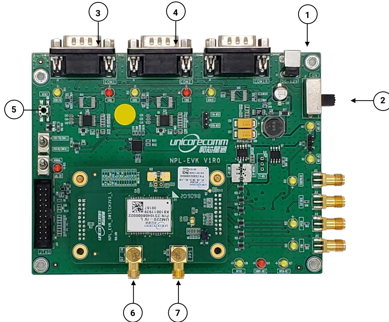
图 2-1 UM220-IV L EVK 板正面图
