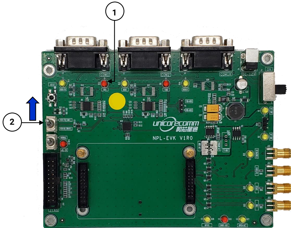
图 2-2 NPL-EVK 板正面图
