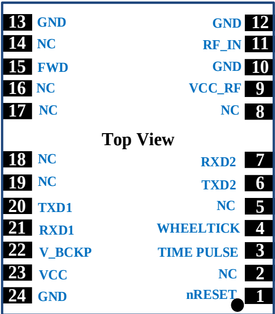
图 3-2 管脚图
