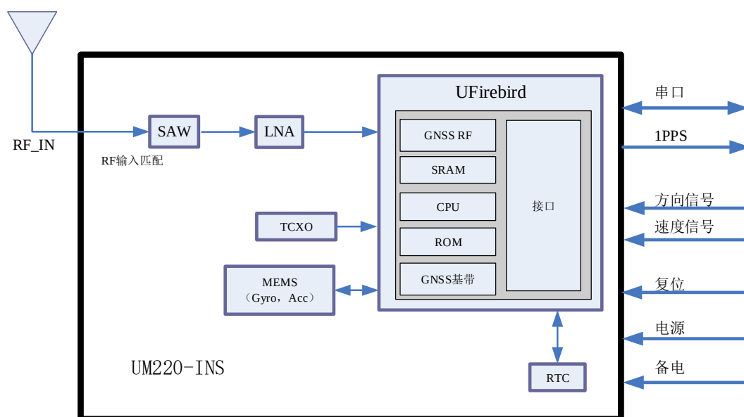
图 1-2 UM220-INS 结构框图
