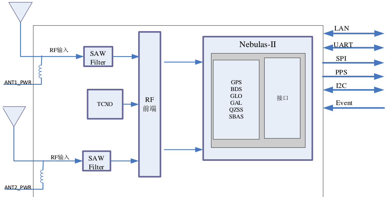
图 1-2 UB482 结构框图
