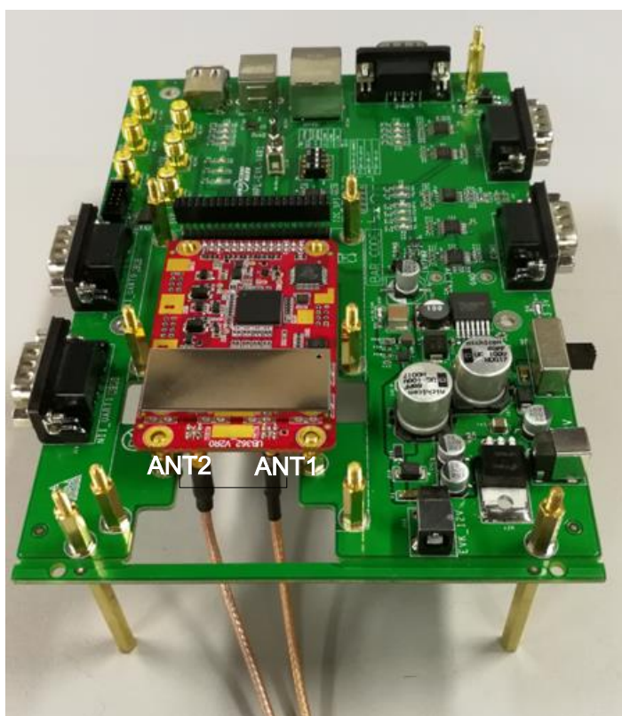
图 4-2 连接天线
